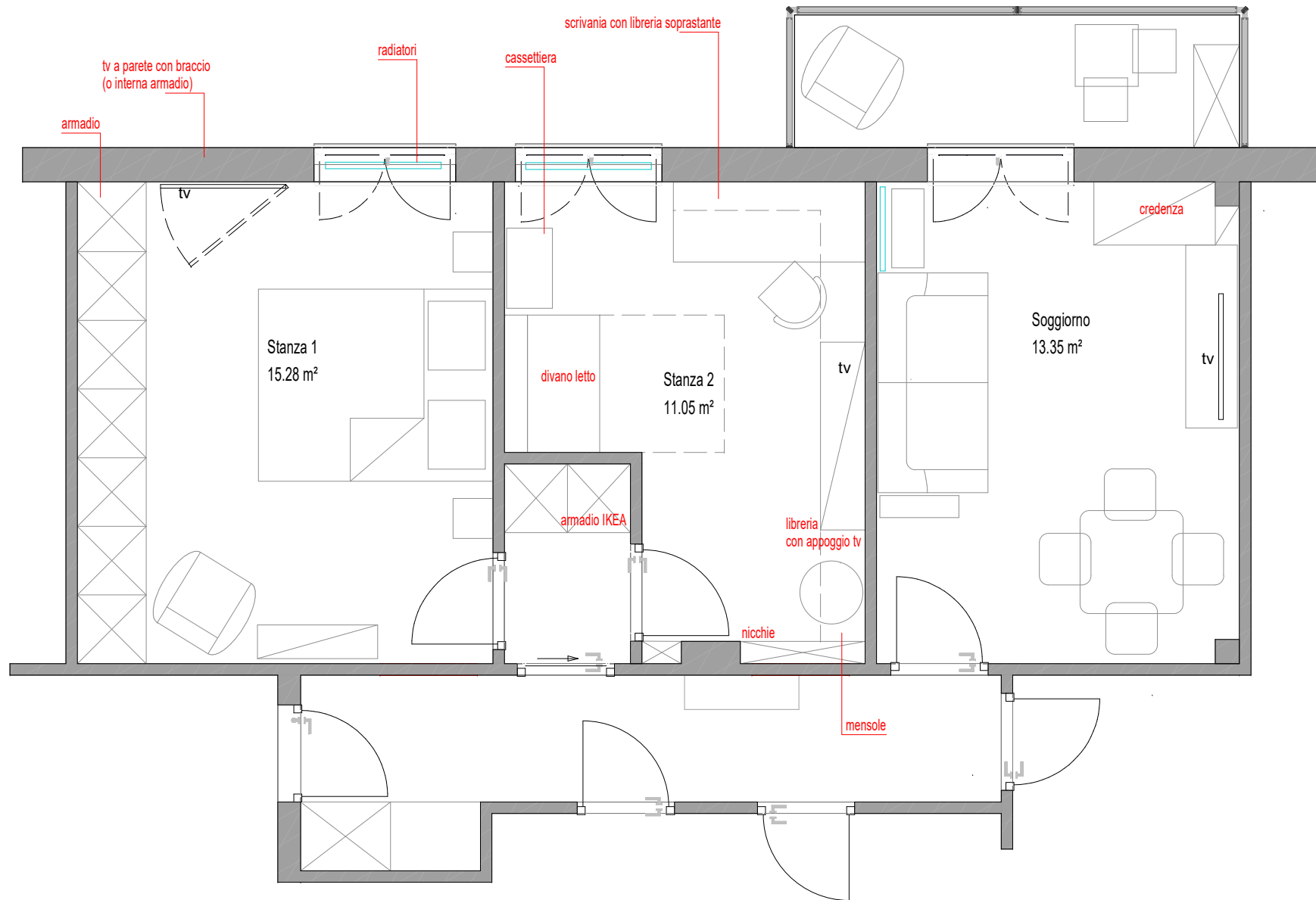
PIANTA DI PROGETTO - SCALA 1:50 -
