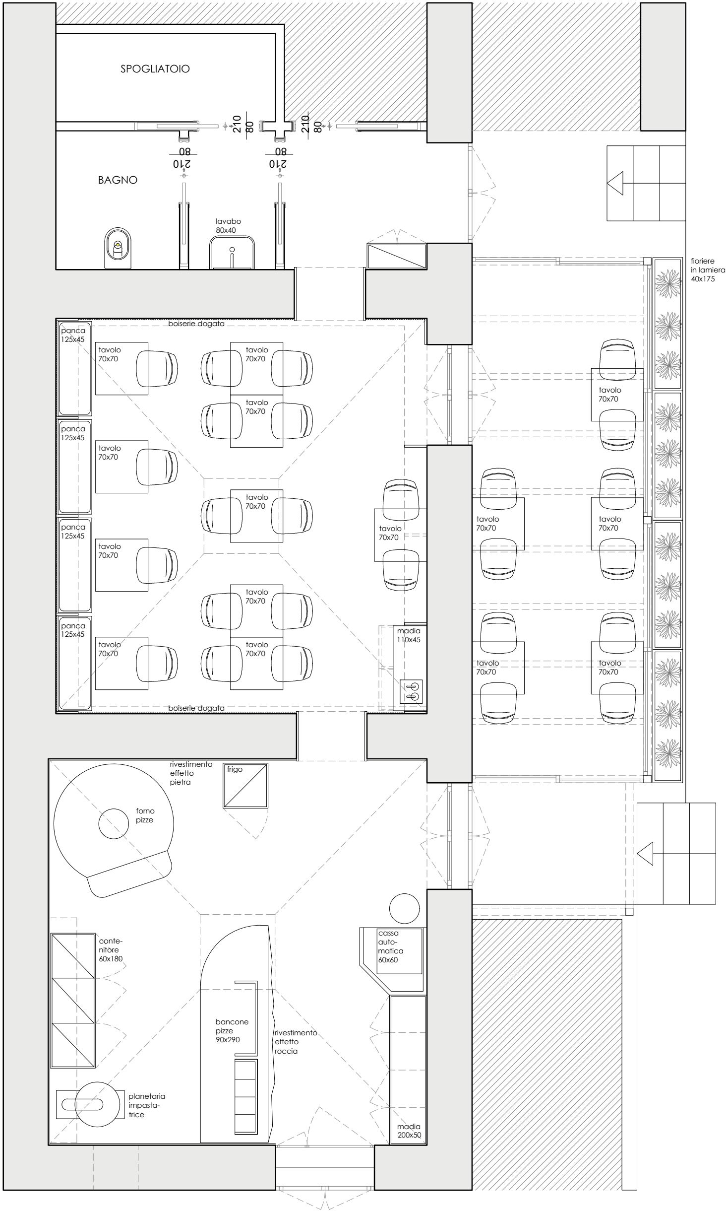
PIANTA PIANO TERRA 60 mq interni + 16 mq esterni coperti
