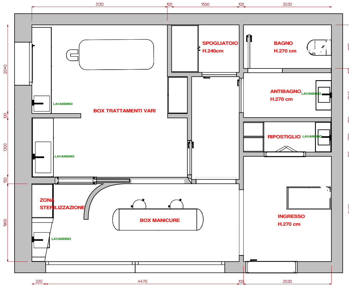
PIANTA CENTRO ESTETICO SCALA 1.20
