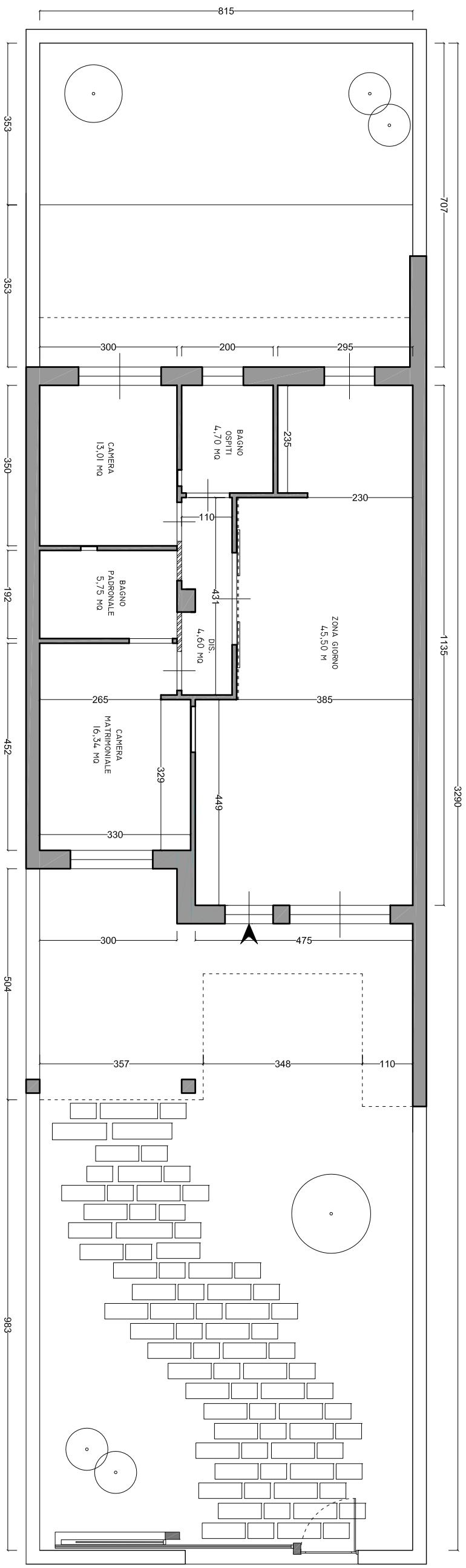
PLANIMETRIA QUOTATA
