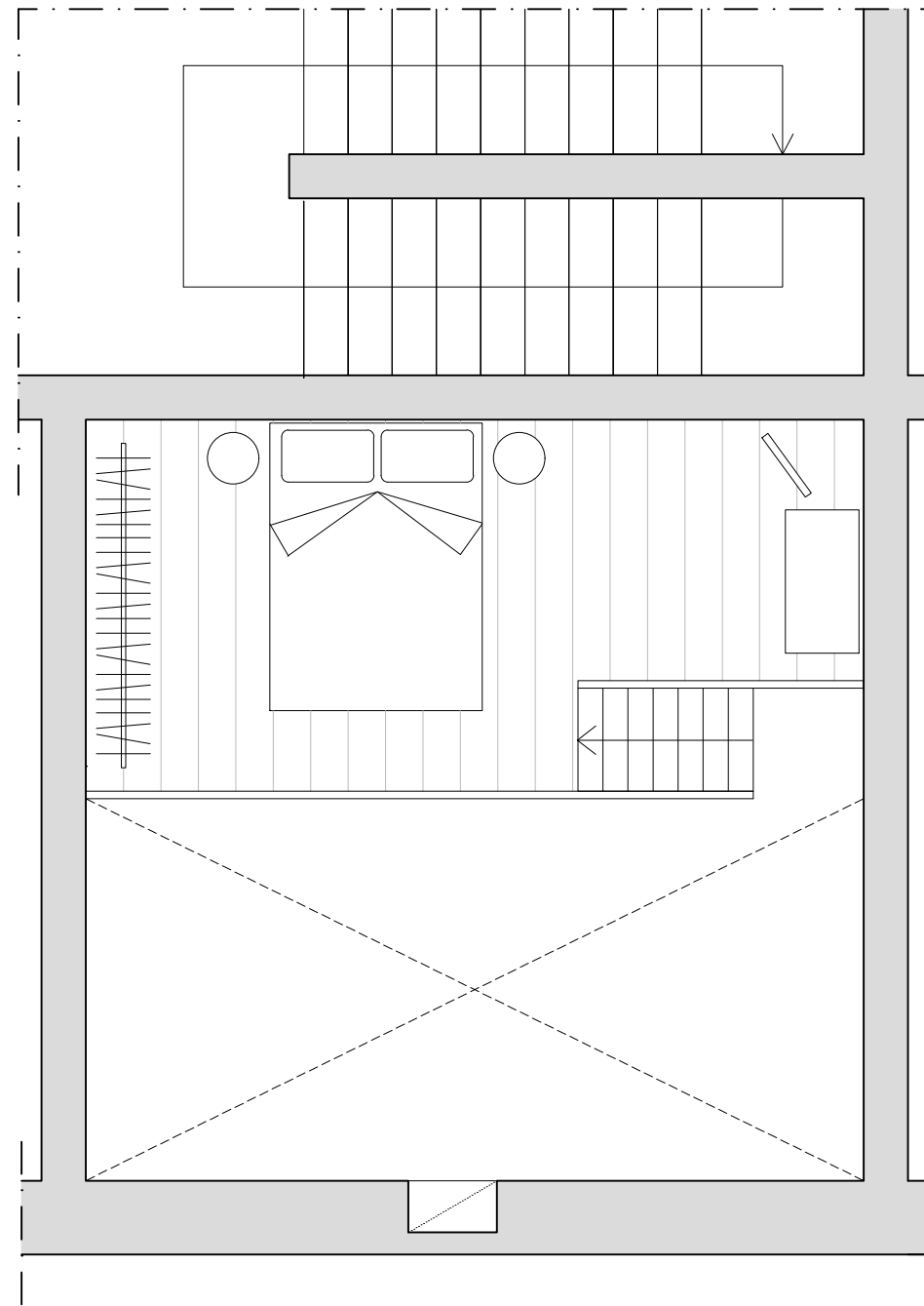
Progetto PIANO SUPERIORE
