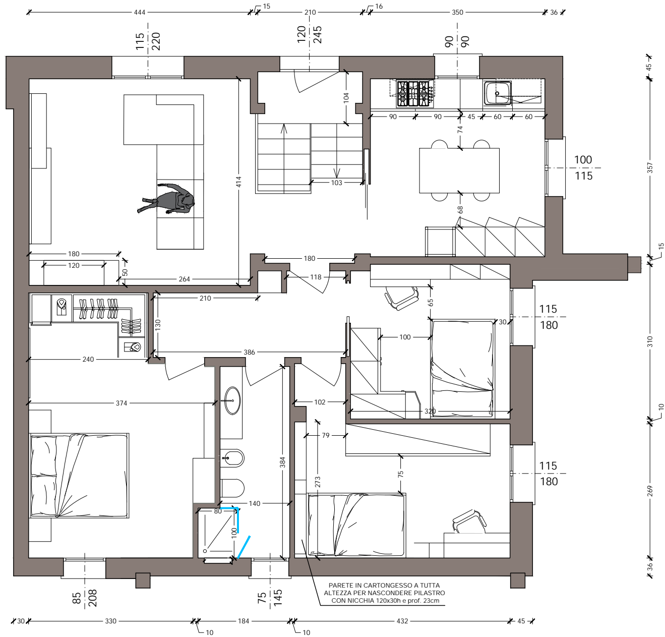
PIANO TERRA - APPARTAMENTO
