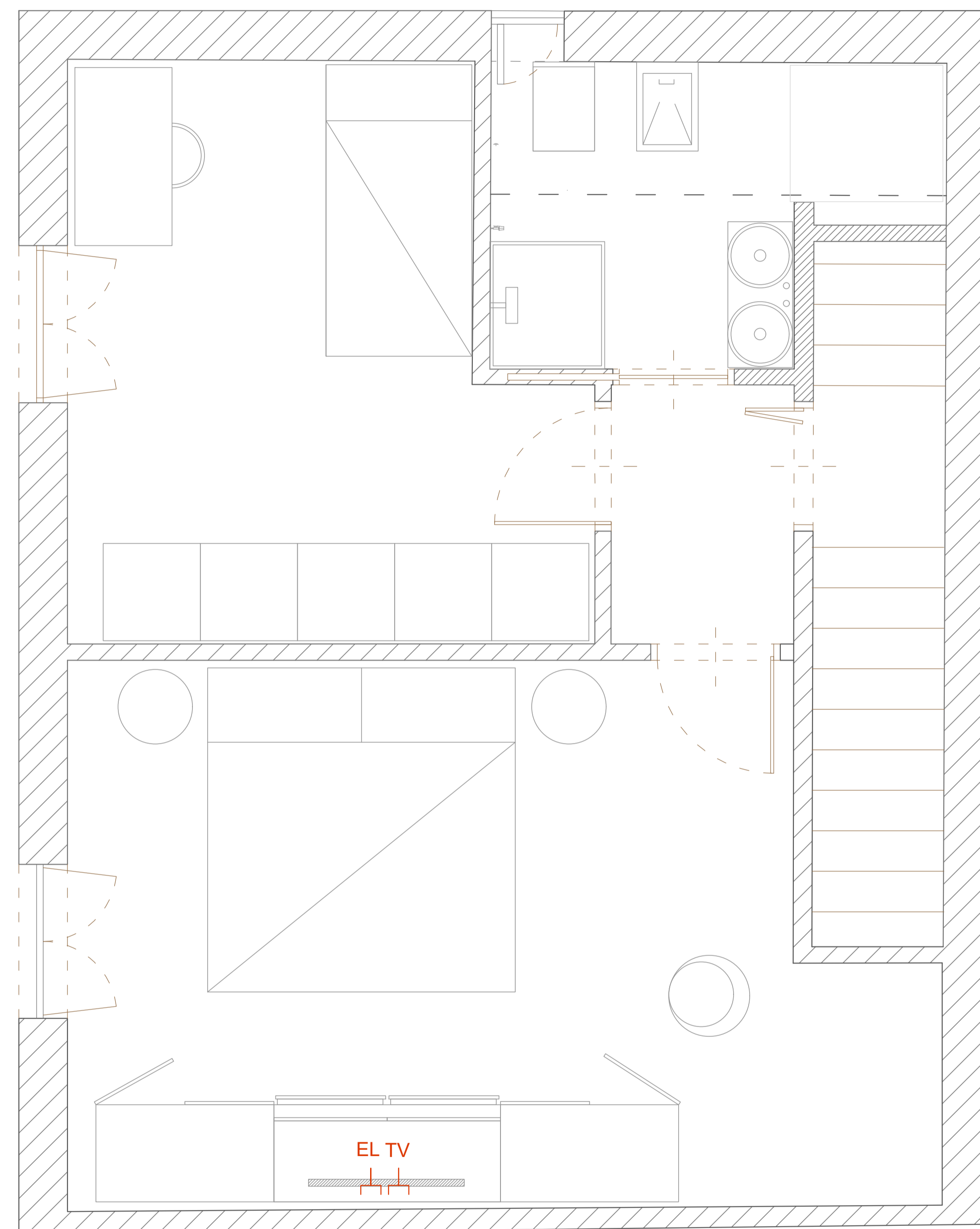
PLANIMETRIA GENERALE - STATO DI PROGETTO h 2,78 mt - SECONDO LIVELLO
