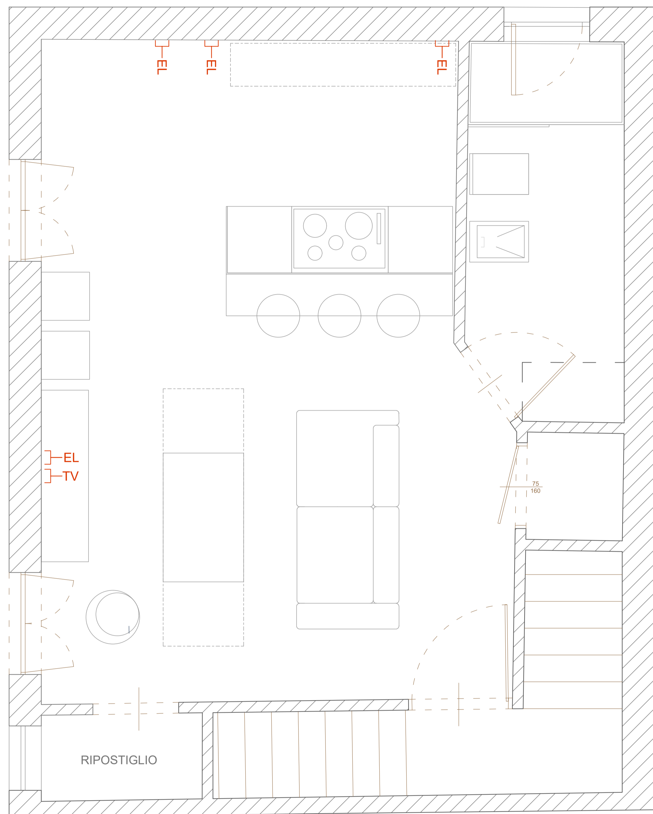
PLANIMETRIA GENERALE - STATO DI PROGETTO h 2,86 mt - PRIMO LIVELLO
