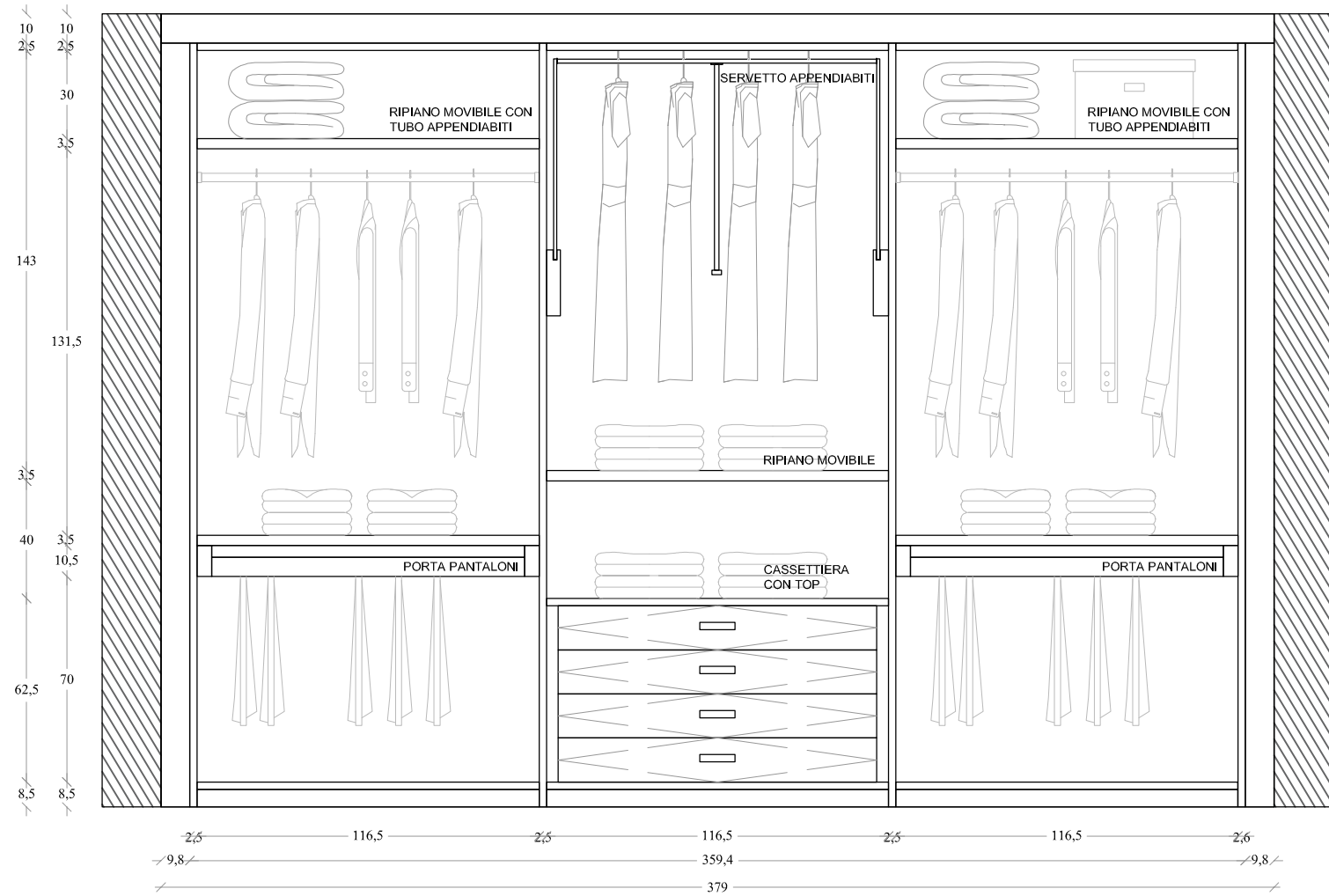
ATTREZZATURA INTERNA
