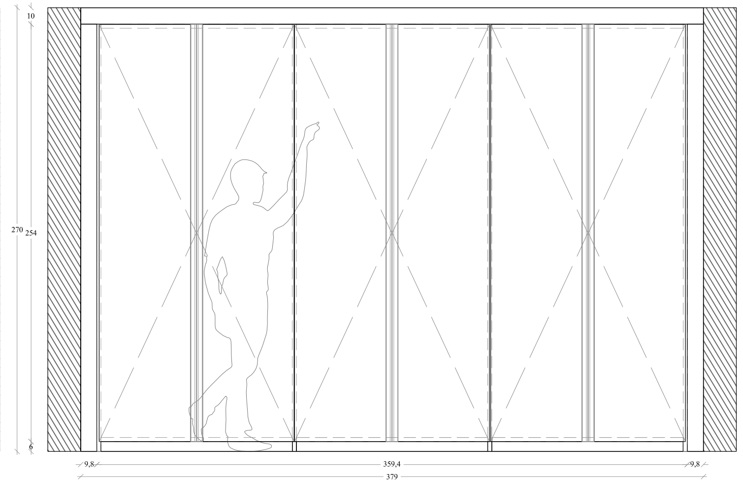
PROSPETTO
