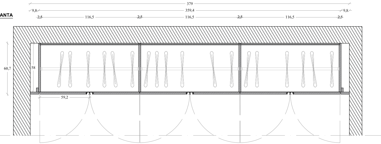
ATTREZZATURA INTERNA
